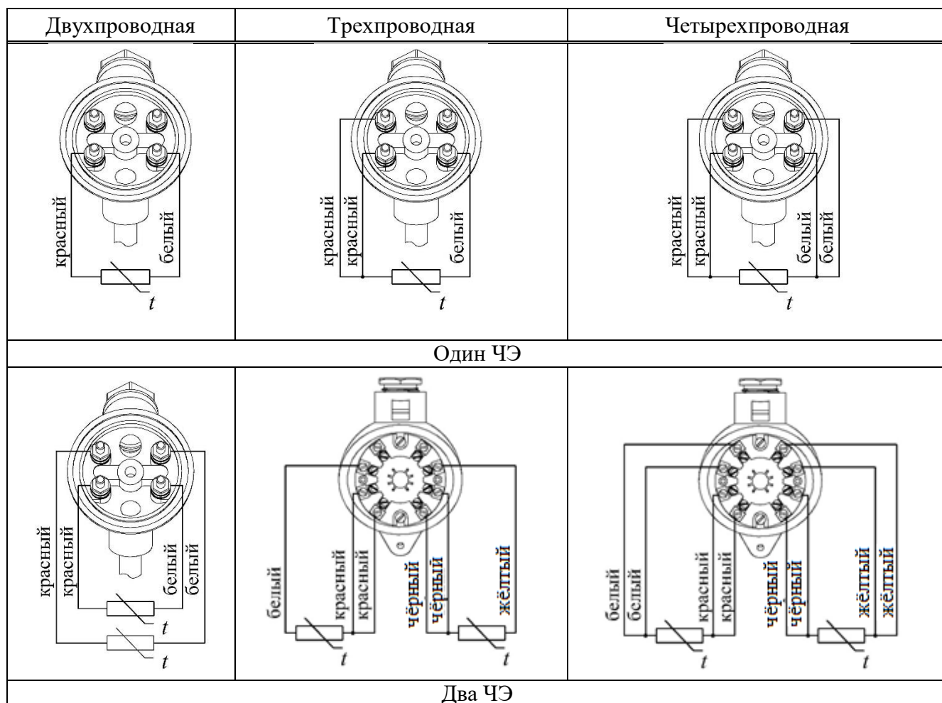
Рис. 2 Схемы подключения проводов к клеммам головок ДТ
